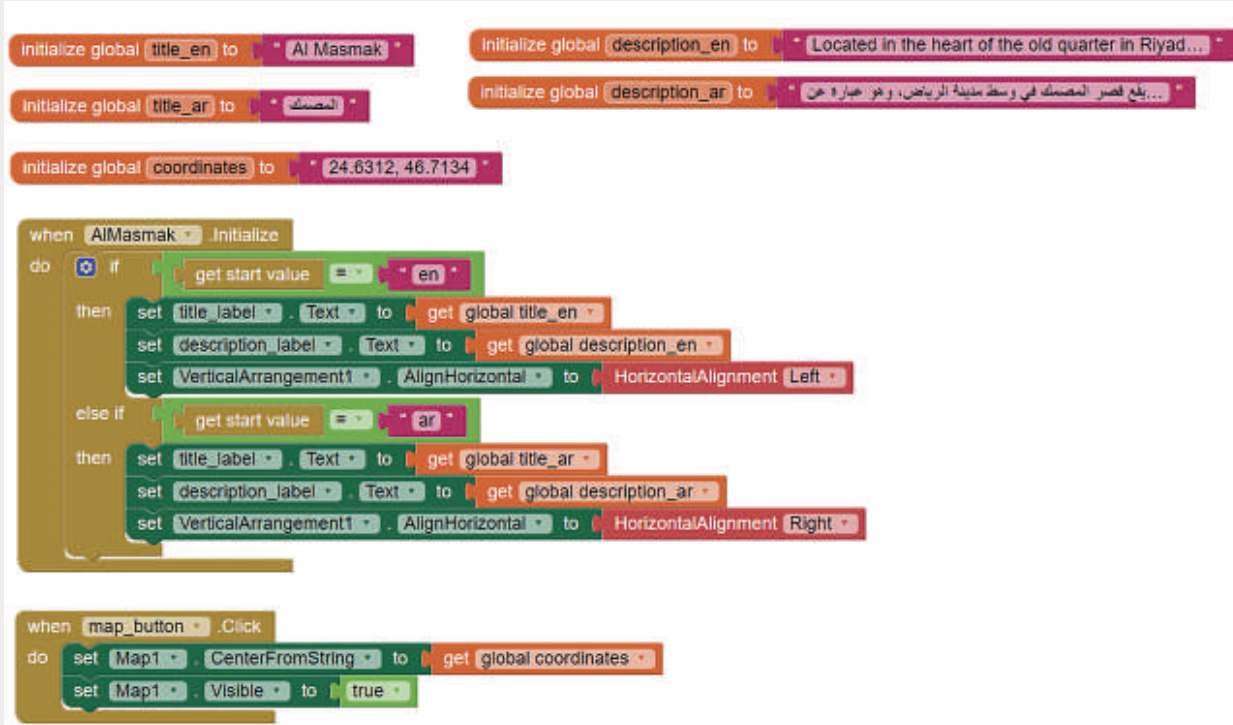
شكل 3.44: البرنامج بشكله النهائي للشاشة الثالثة
