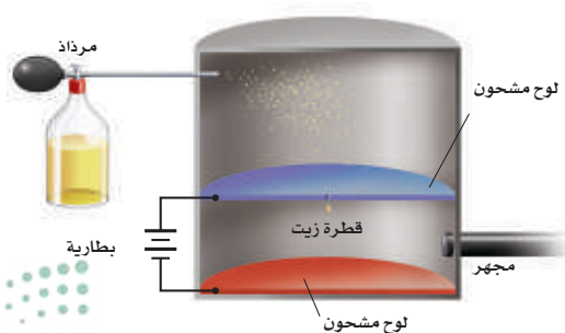
الشكل 9-10 يوضح هذا الشكل مقطّعاً عرضياً للجهاز الذي استخدمه مليكان في حساب شحنة الإلكترون.
