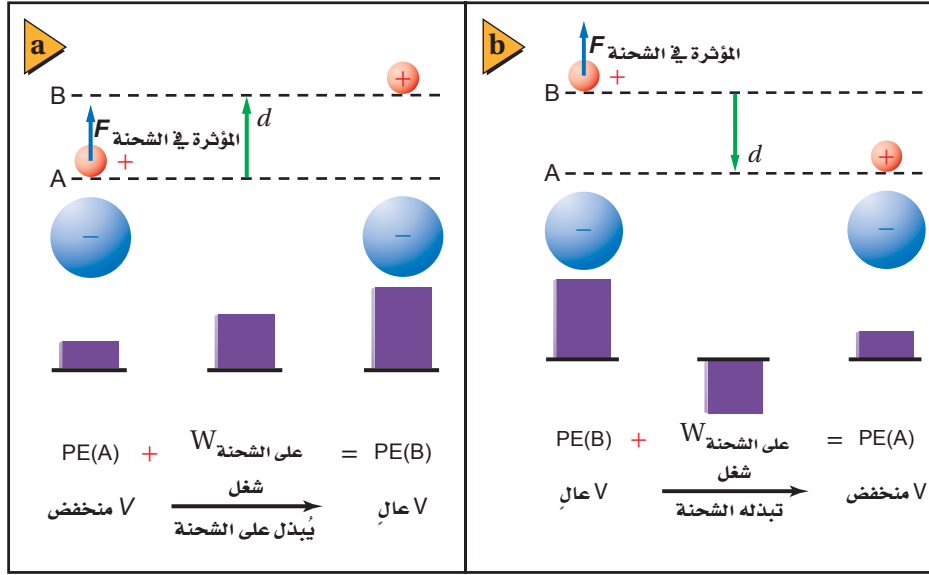
■ الشكل 9-6 يُحسب فرق الجهد الكهربائي من خلال قياس الشغل المبذول لكل وحدة شحنة. يزداد فرق الجهد الكهربائي عند إبعاد الشحنات المختلفة بعضها عن بعض (a). ويقل فرق الجهد الكهربائي عند تقريب الشحنات المختلفة بعضها إلى بعض (b).
