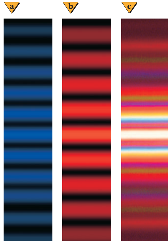
■ الشكل 2-7 أنماط تداخل الشقّ المزدوج للضوء الأزرق (a)، وللضوء الأحمر (b)، وللضوء الأبيض (c).
