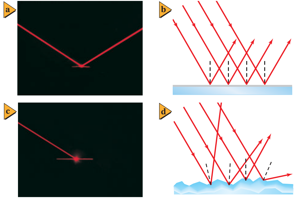
■ الشكل 3-5 عندما تسقط حزمة ضوئية على سطح مرآة (a) تنعكس الأشعة المتوازية في الحزمة الساقطة متوازيةً ومحافظةً على شكل الحزمة (b). وعندما تسقط حزمة الضوء على سطح خشن (c) تنعكس الأشعة المتوازية في الحزمة الساقطة عن سطوح مختلفة صغيرة جداً، مما يؤدي إلى تشتيت الأشعة (d).
