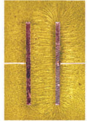
الشكل 9-9 تمثيل لمجال كهربائي بين لوحين متوازيين.
