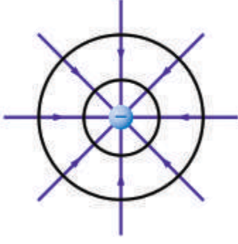
■ الشكل 7-9 فرق الجهد الكهربائي بين أي نقطتين على أي مسار دائري حول شحنة يساوي صفر.
