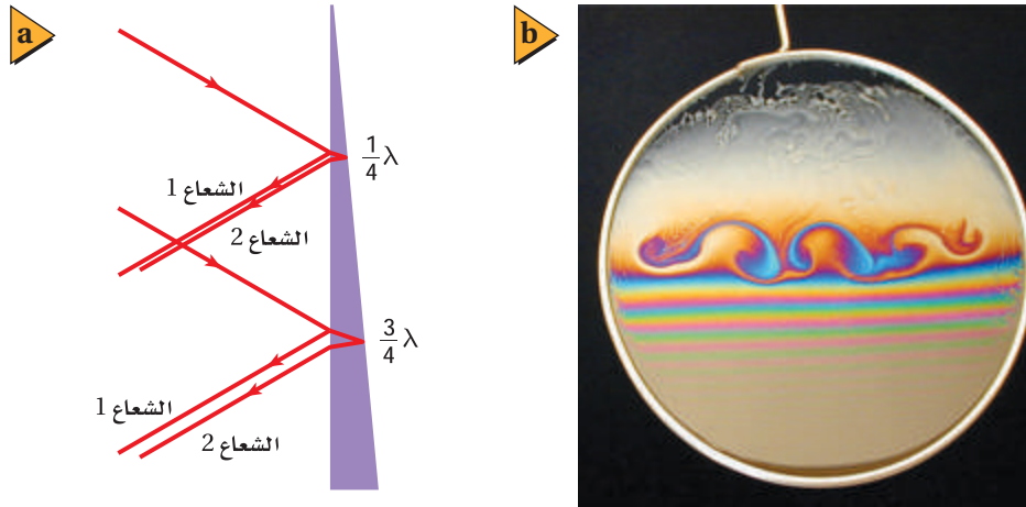
■ الشكل 6-7 يحدث تقوية لكل طول موجي عندما يكون سُمك غشاء الصابون \lambda/4 ، 3\lambda/4 ، 5\lambda/4 (a). ولأن كل لون له طول موجي خاص به فإن سلسلة الأهداب التي تنعكس عن غشاء الصابون تكون ملونة (b).
