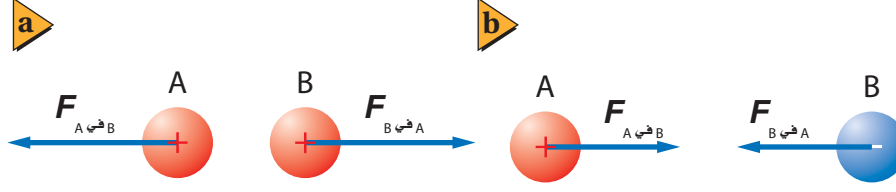
■ الشكل 8-13 قاعدة تحديد اتجاه القوة هي: الشحنات المتشابهة تتنافر؛ والشحنات المختلفة تتجاذب.
