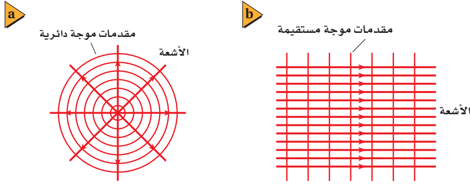
■ الشكل 1-7 تتولد مقدمات موجات الضوء المنتظمة من المصادر النقطية (a)، وأشعة الليزر (b).
