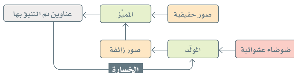
شكل 4.28: معمارية الشبكة التوليدية التنافسية
