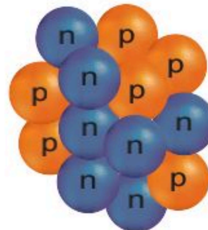
نواة ذرة كربون - ١٣
