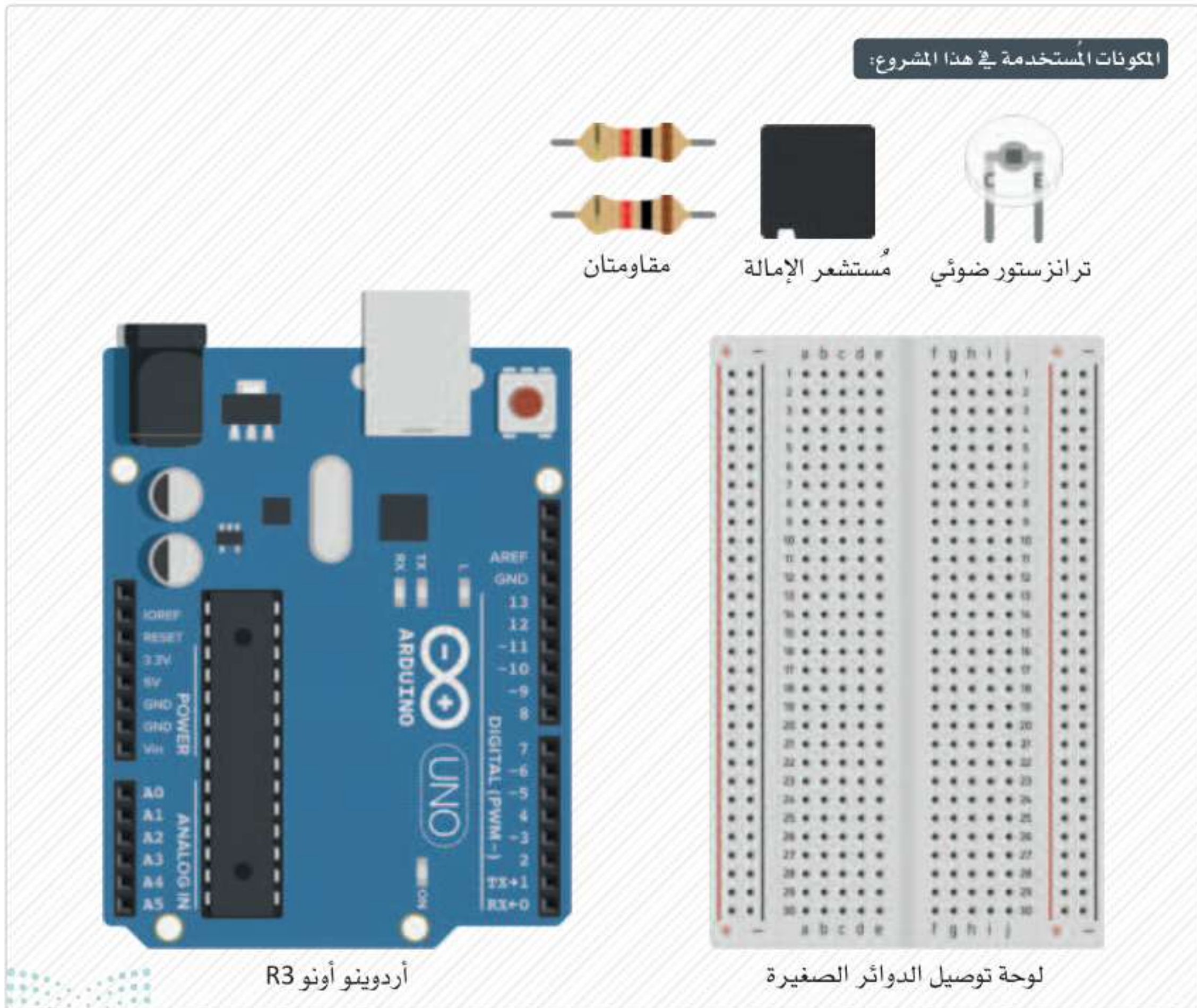
شكل 7.11: مكونات مشروع النفايات الذكية
