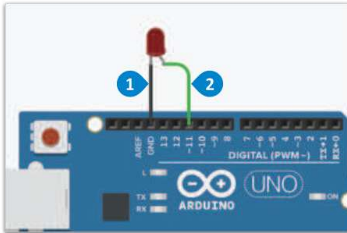
شكل 6.12: توصيل الدايود المشع للضوء
