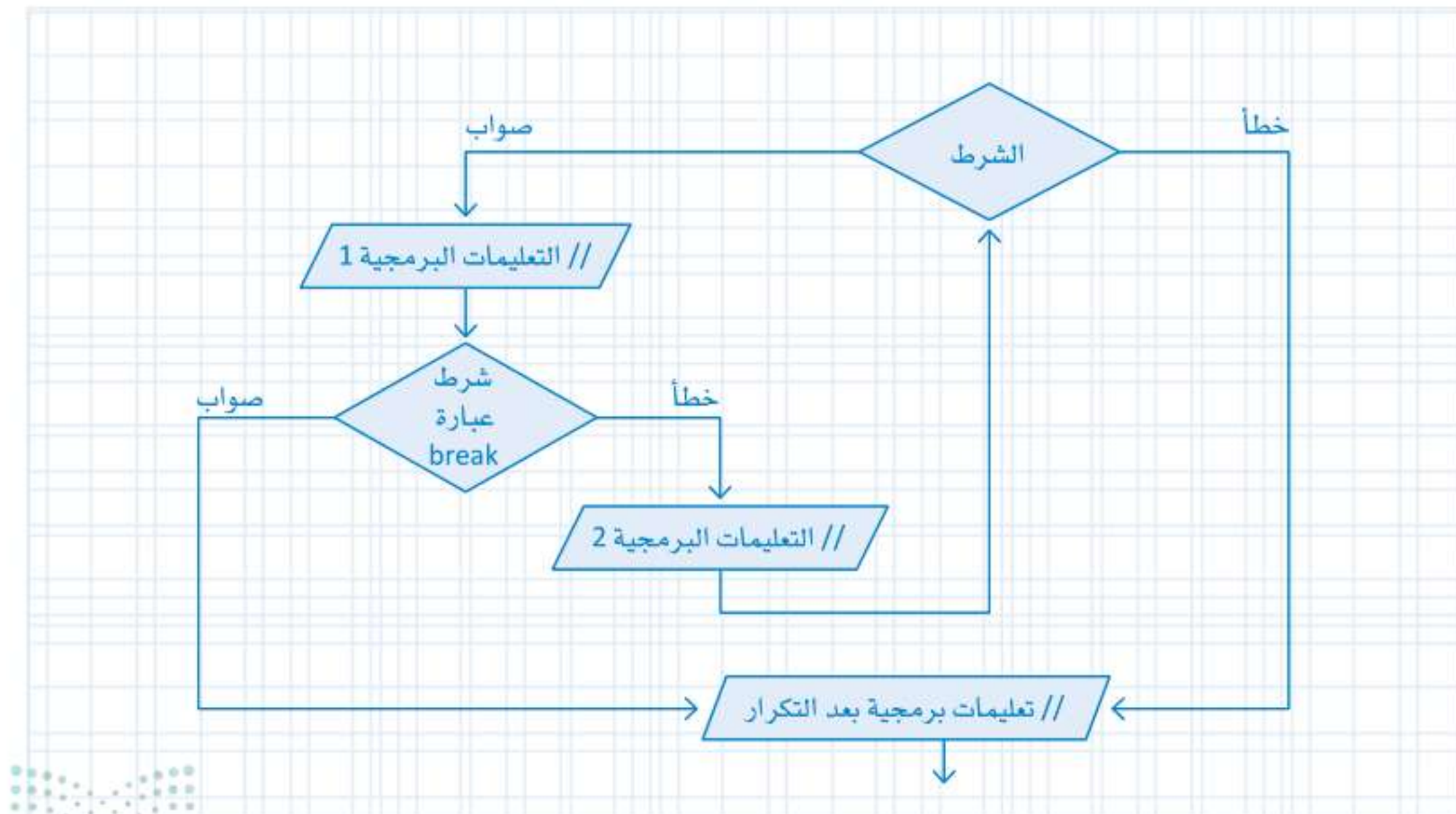
شكل 6.8: مخطط عبارة break
