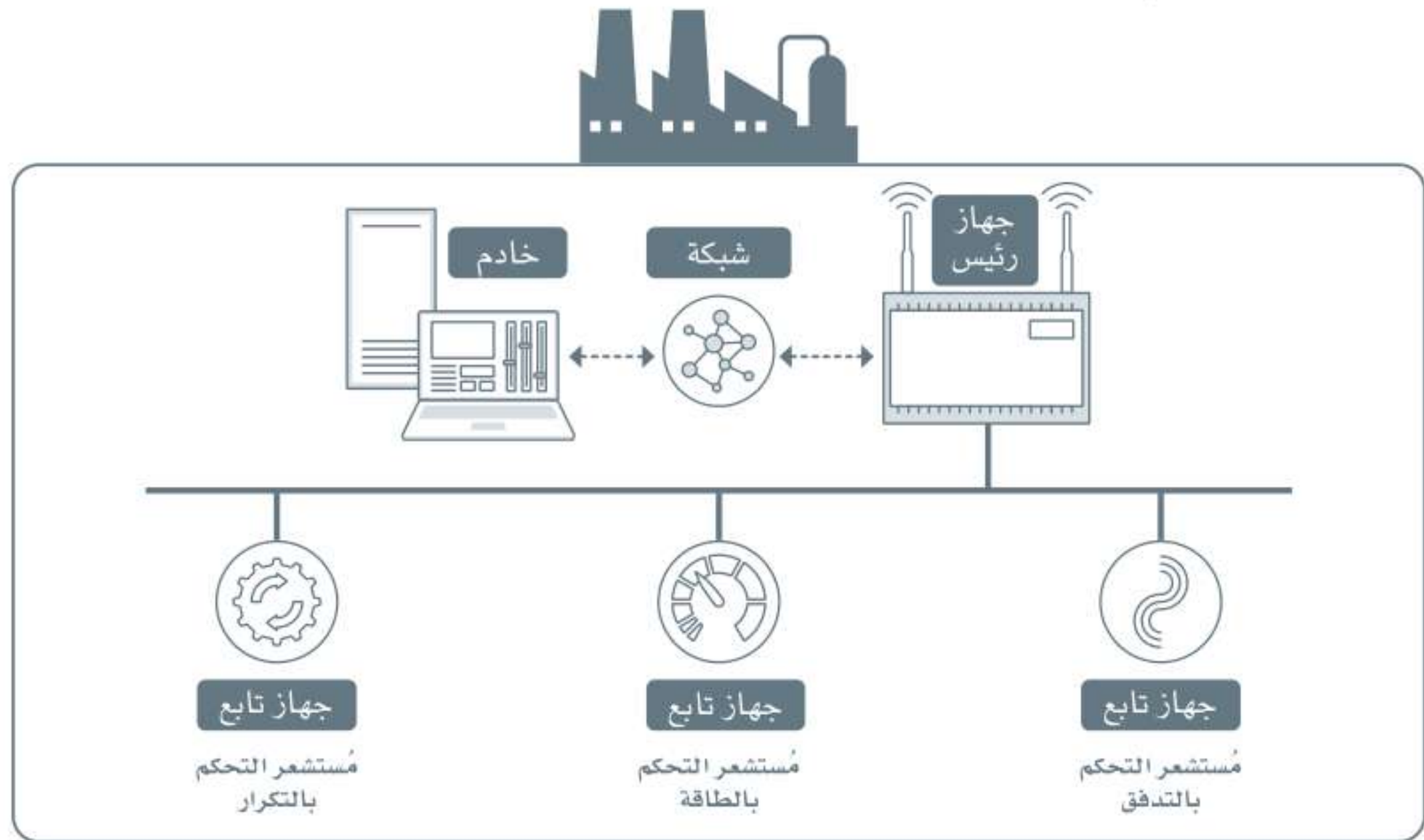
شكل 8.1: بروتوكول الشبكة مودبس (Modbus)
