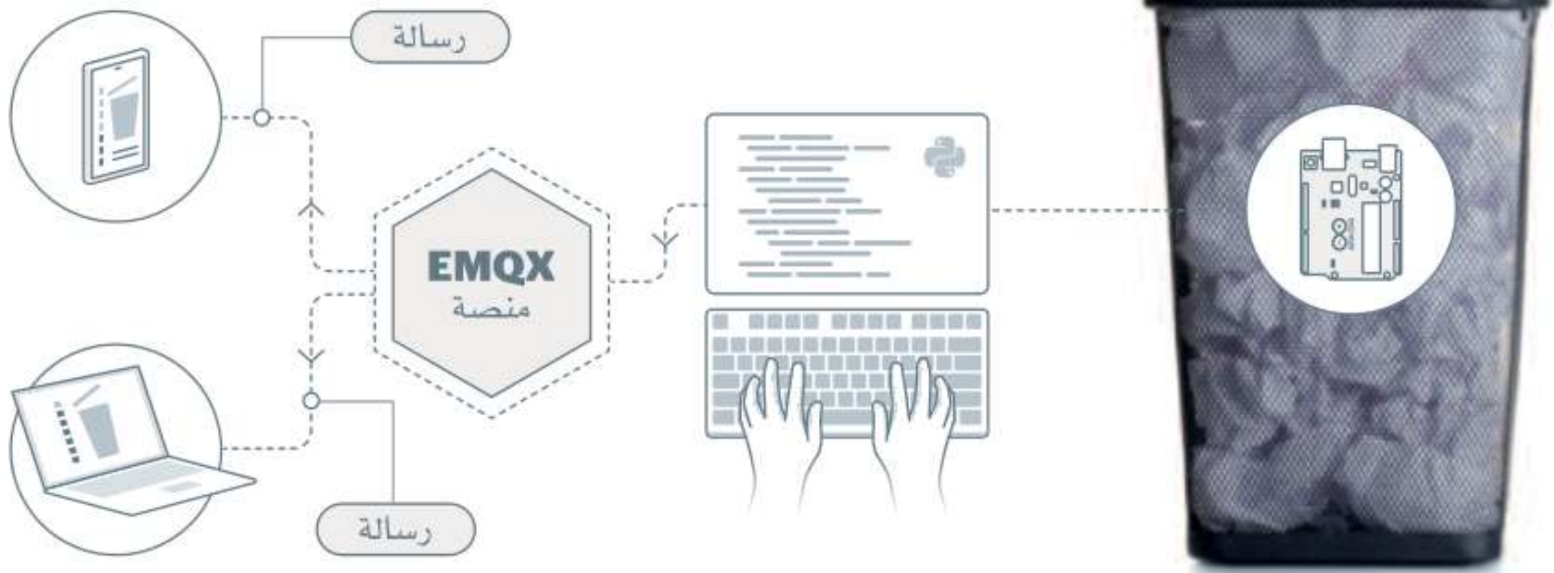
شكل 7.8: مشروع إدارة النفايات الذكية بالأردوينو وبروتوكول MQTT
