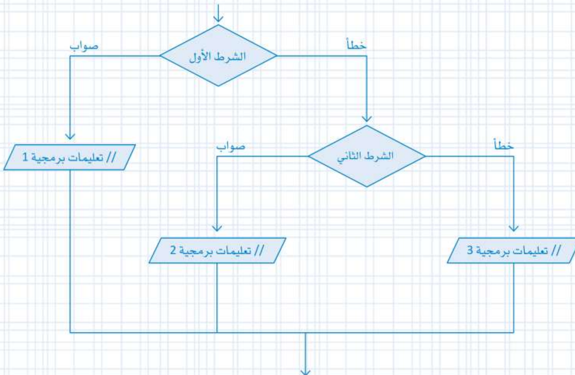
شكل 6.4: مخطط عبارة if .. else if .. else
