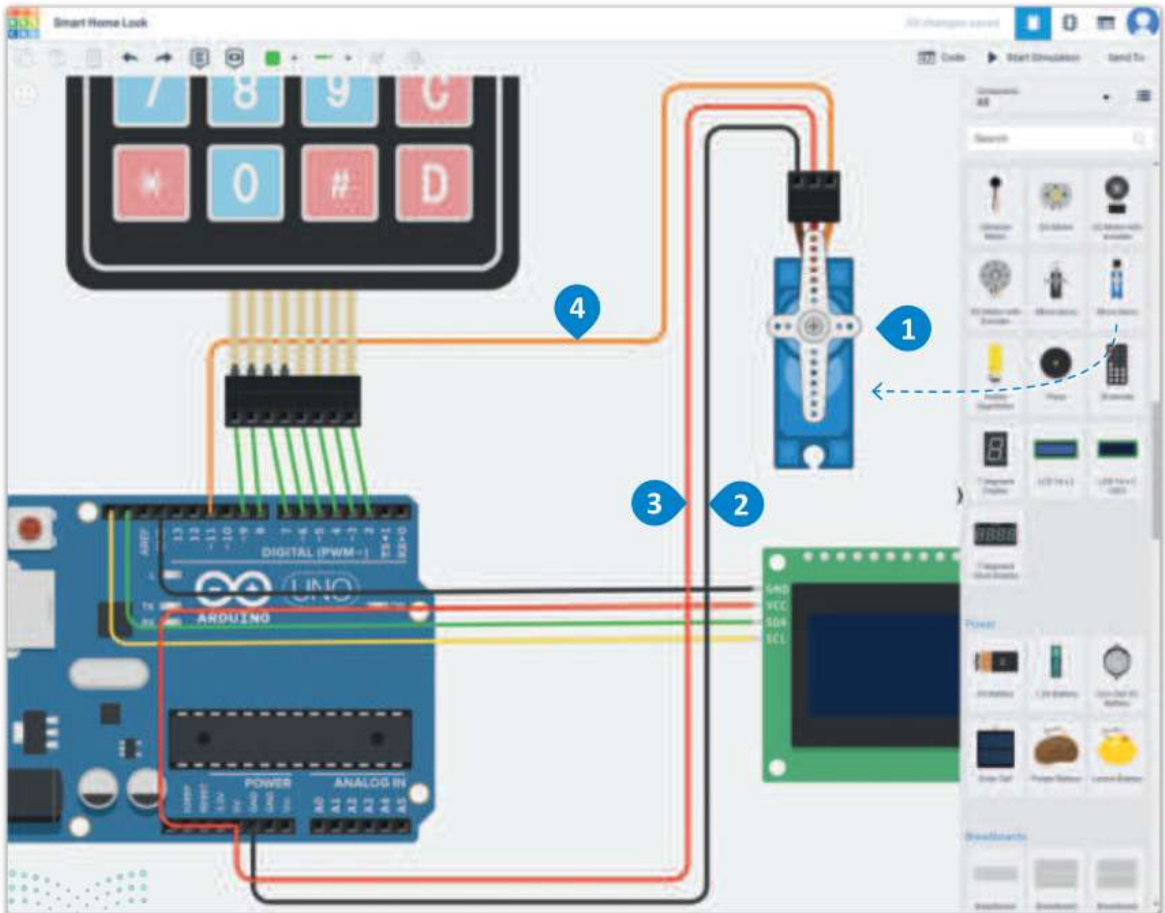
شكل 6.20: توصيل محرك السيرفو المصغر
