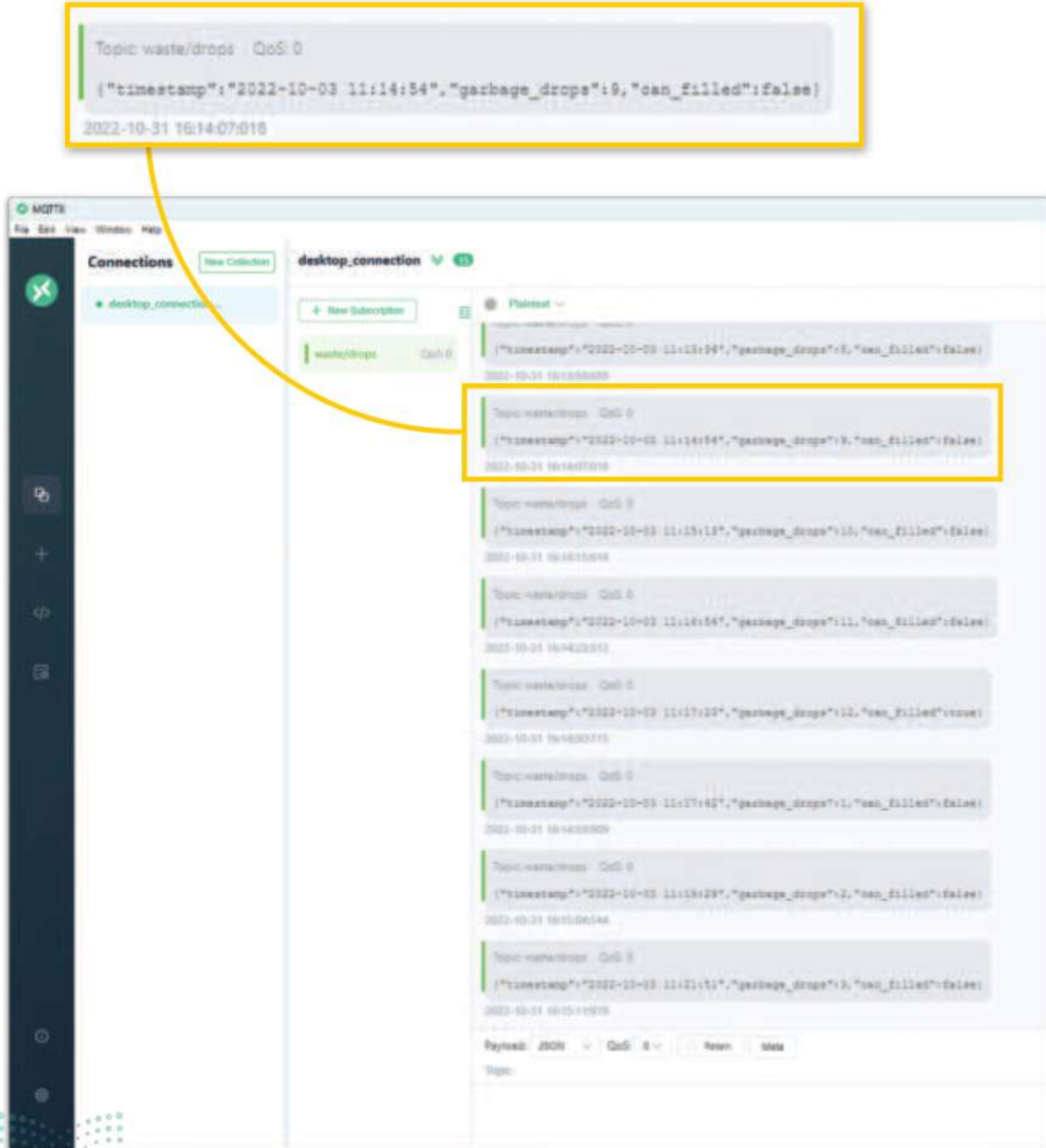
شكل 7.20: عرض الرسائل من خلال عميل MQTTX
