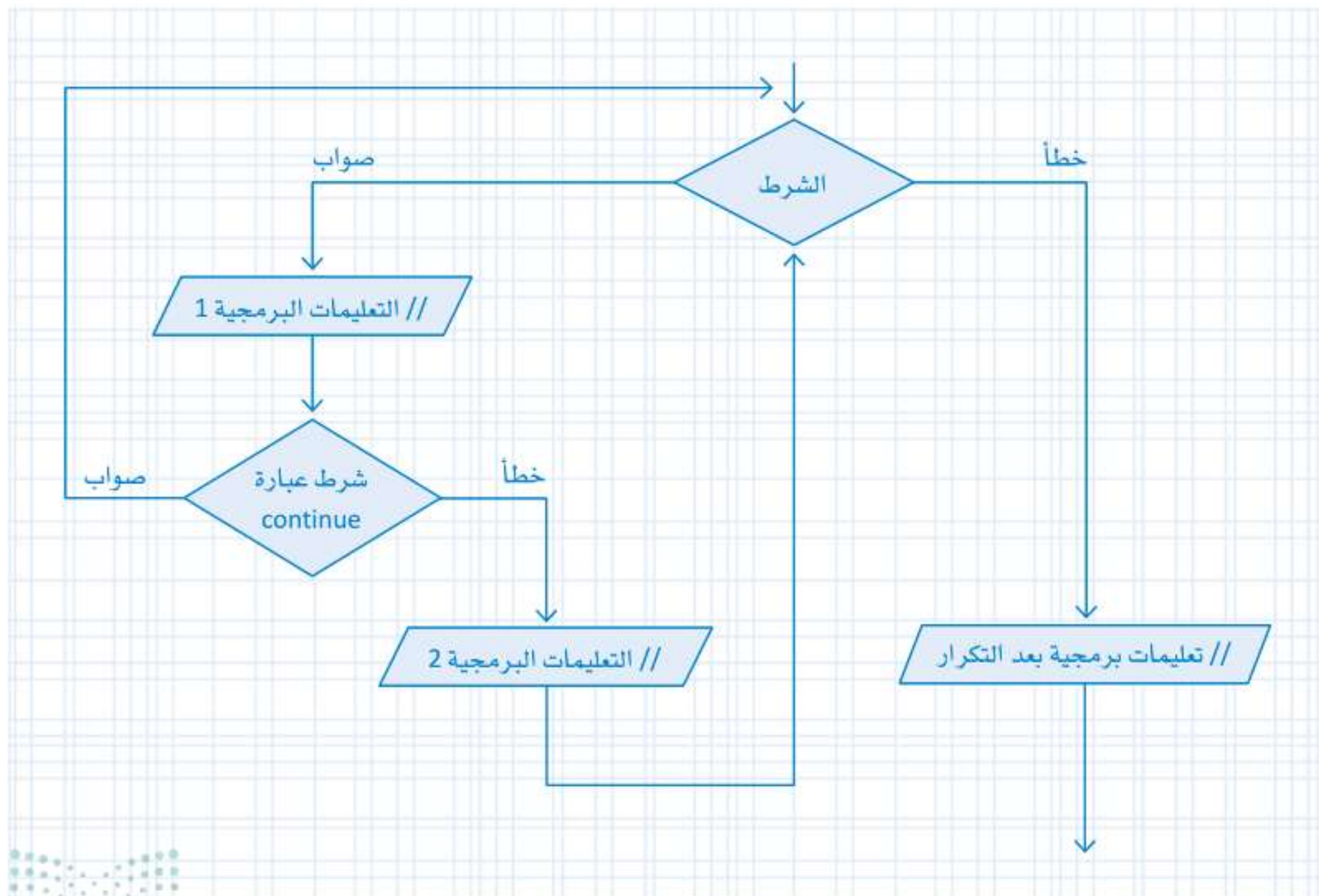
شكل 6.9: مخطط عبارة continue
