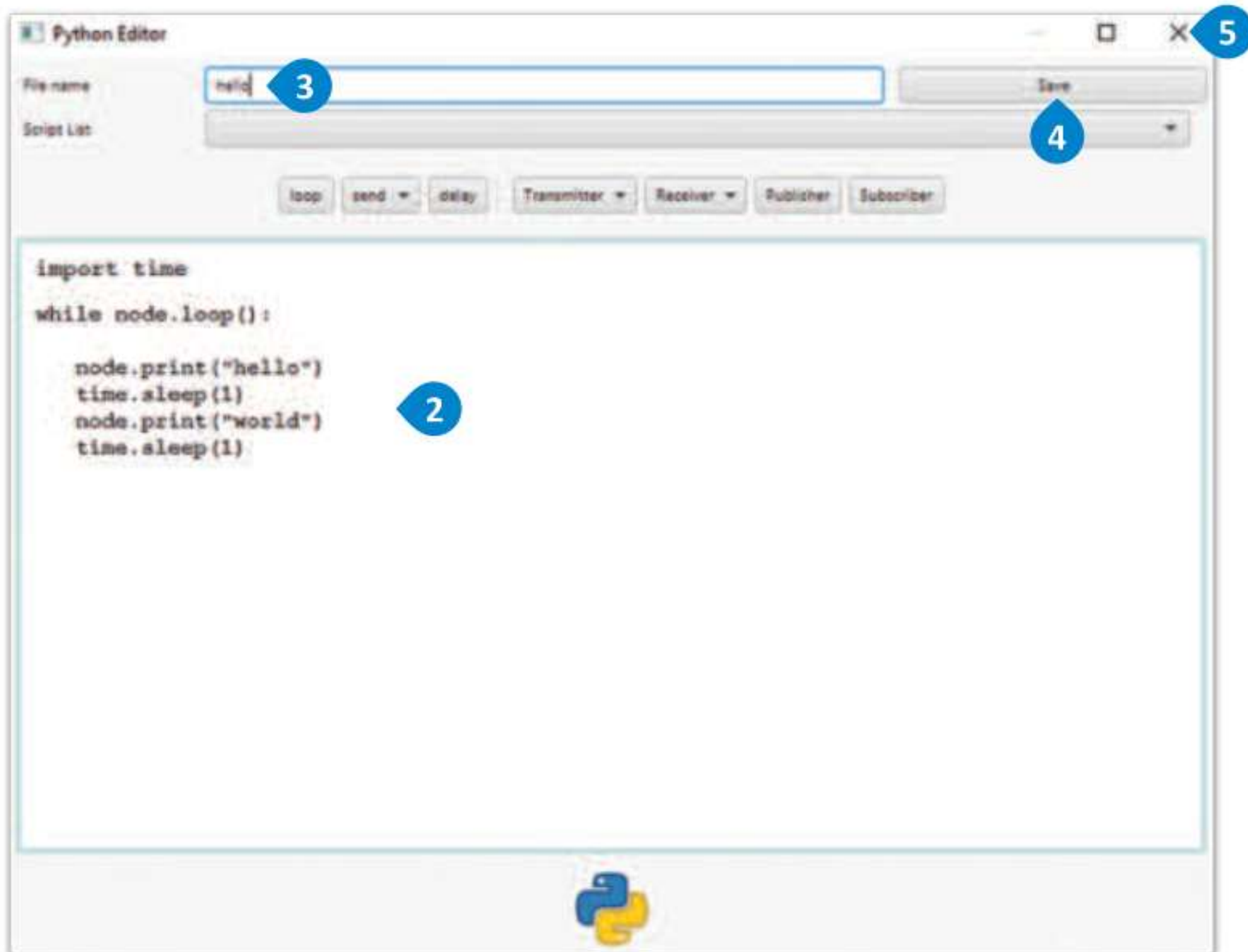
شكل 8.9: مُحرر البايثون
