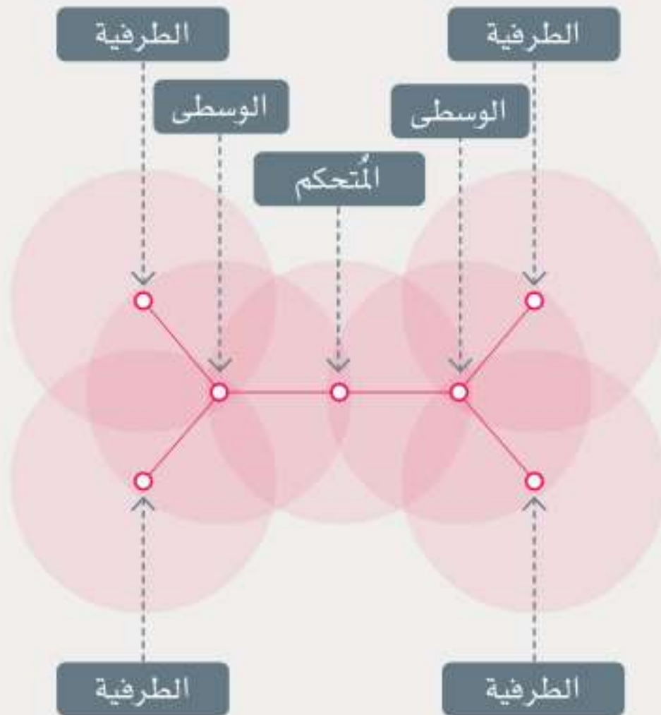
شكل 8.12: العقد ووظائفها
