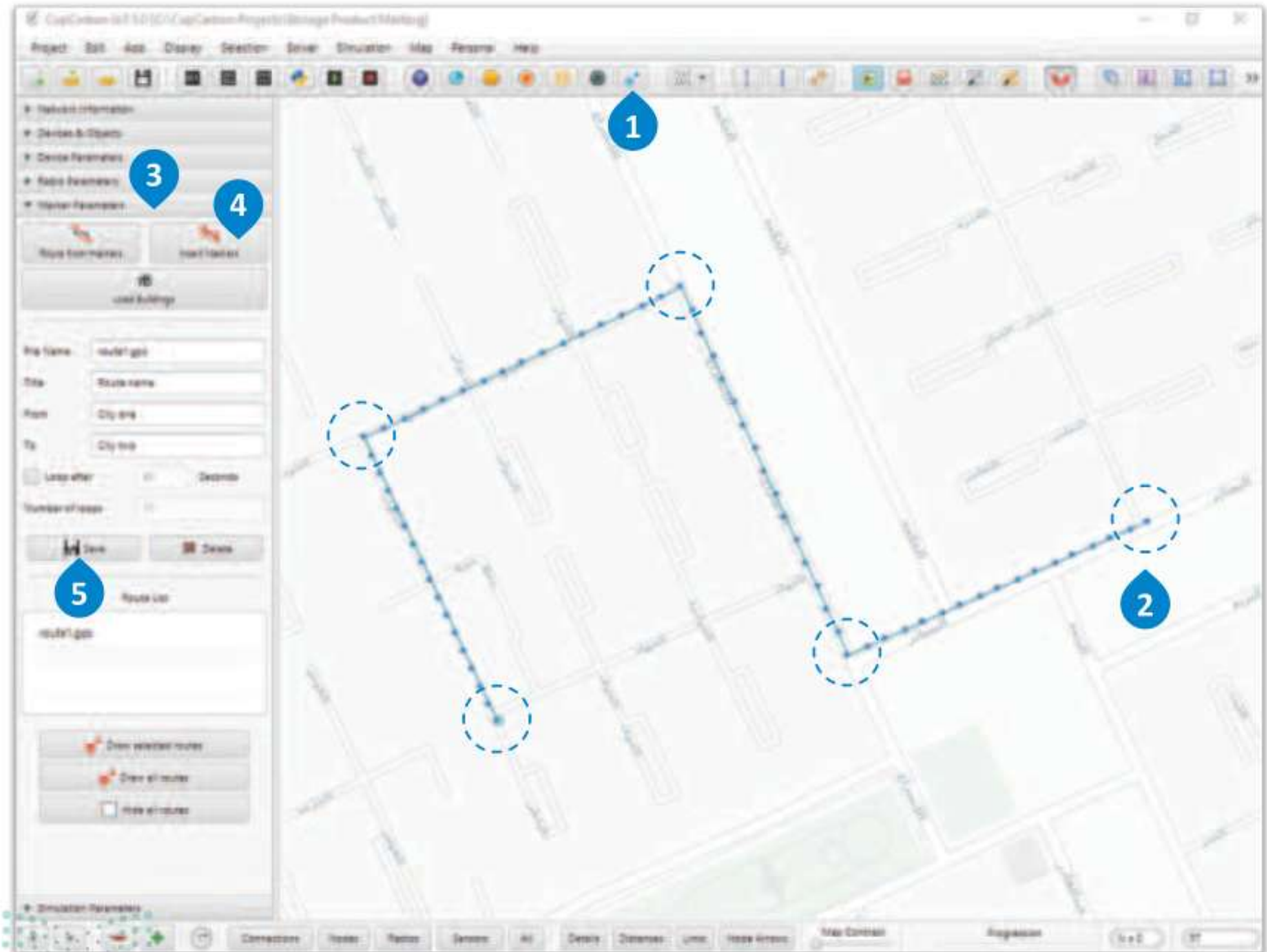
شكل 8.22: إنشاء مسار
