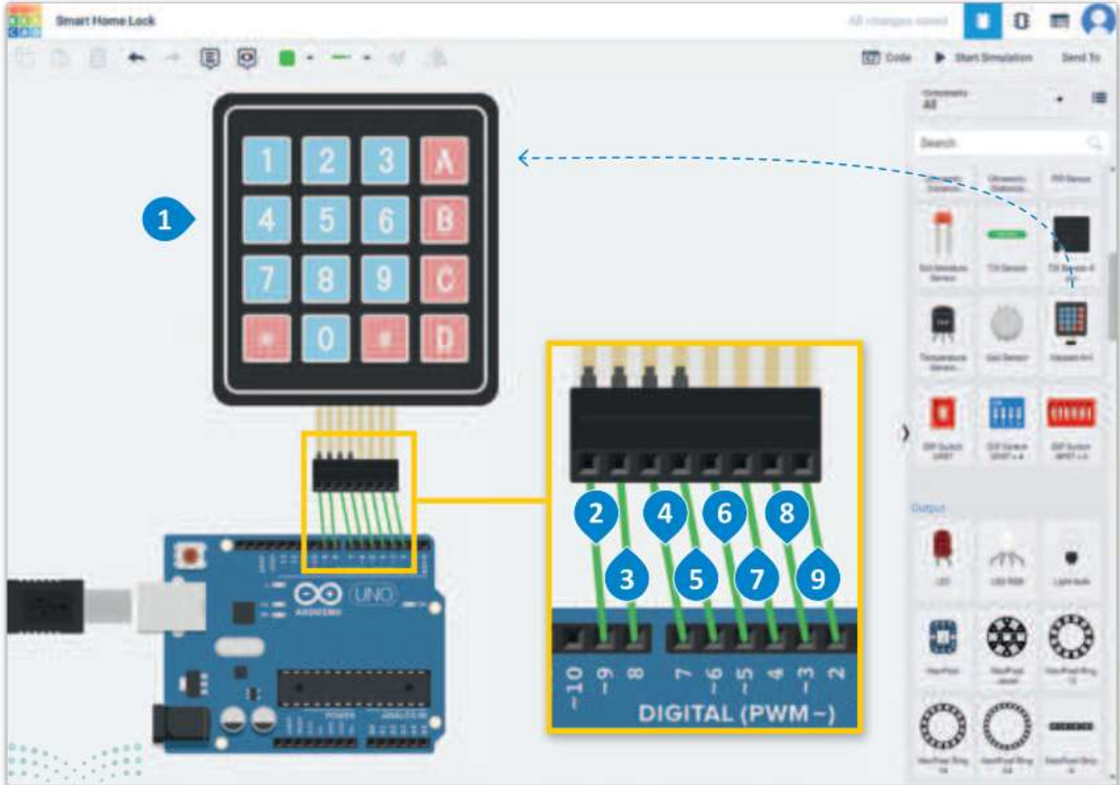
شكل 6.18: توصيل لوحة المفاتيح
