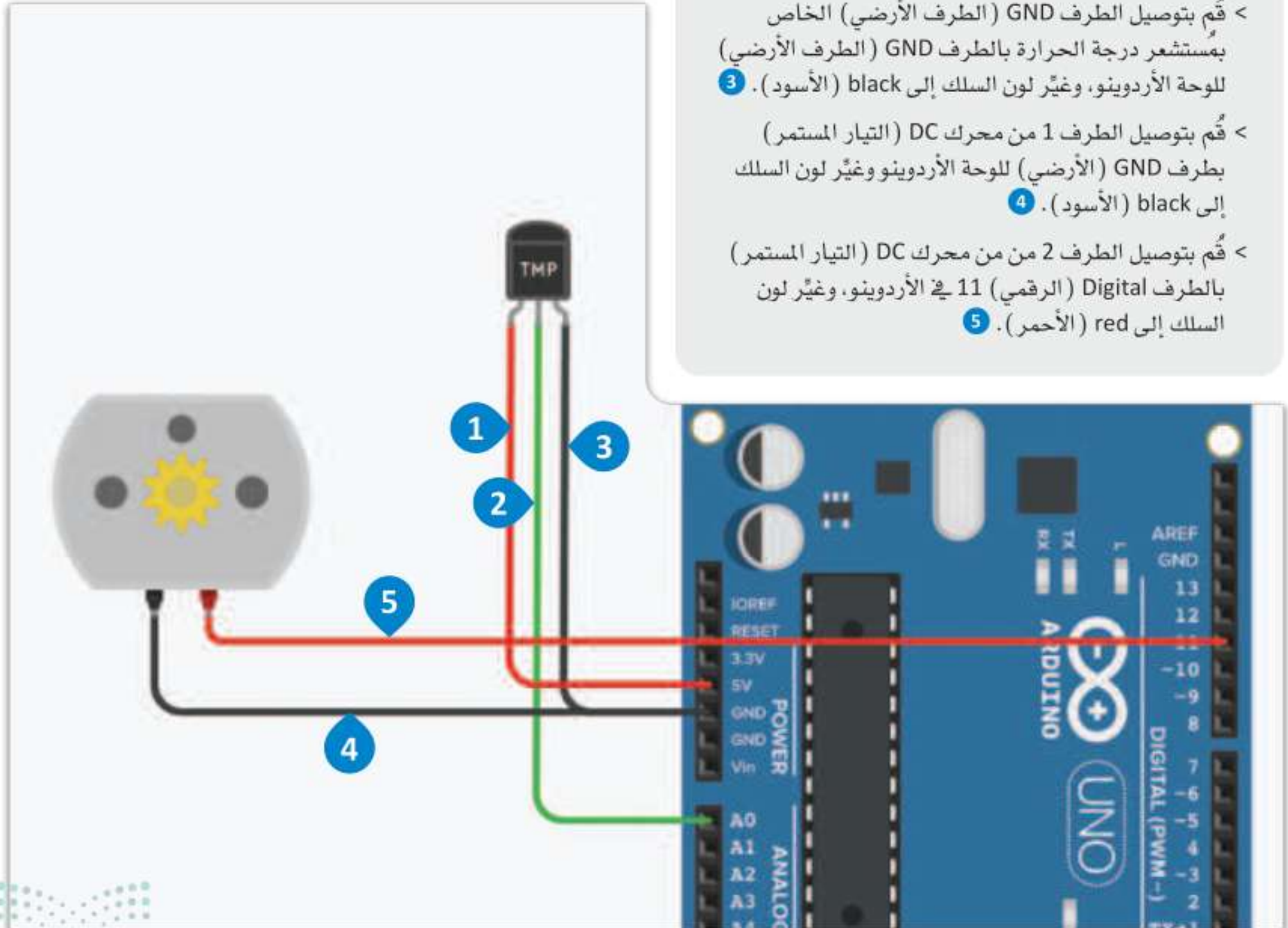
شكل 6.16: توصيل الدائرة
