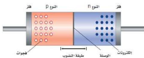
وصلة الدايدود
